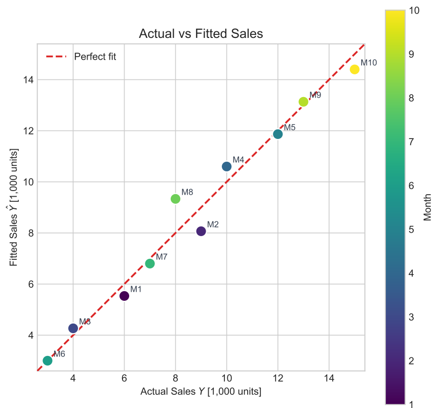
รูปที่ 3: Actual vs Fitted Sales — จุดทุกจุดอยู่ใกล้เส้น Perfect Fit ( Y = \hat{Y} ) ด้านแดงพระ แสดงว่าโมเดล fit ข้อมูลได้ดี
