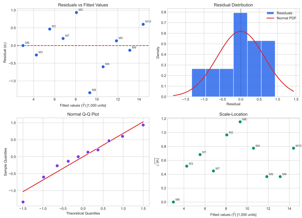
รูปที่ 2: Residual Diagnostics Panel — (top-left) Residuals vs Fitted แสดงว่า residuals ไม่มีรูปแบบชัดเจนรอบเส้นศูนย์; (top-right) Residual Distribution การกระจายใกล้เคียง Normal; (bottom-left) Q-Q Plot ยืนยันความเป็น Normal; (bottom-right) Scale-Location ไม่พบ Heteroscedasticity
